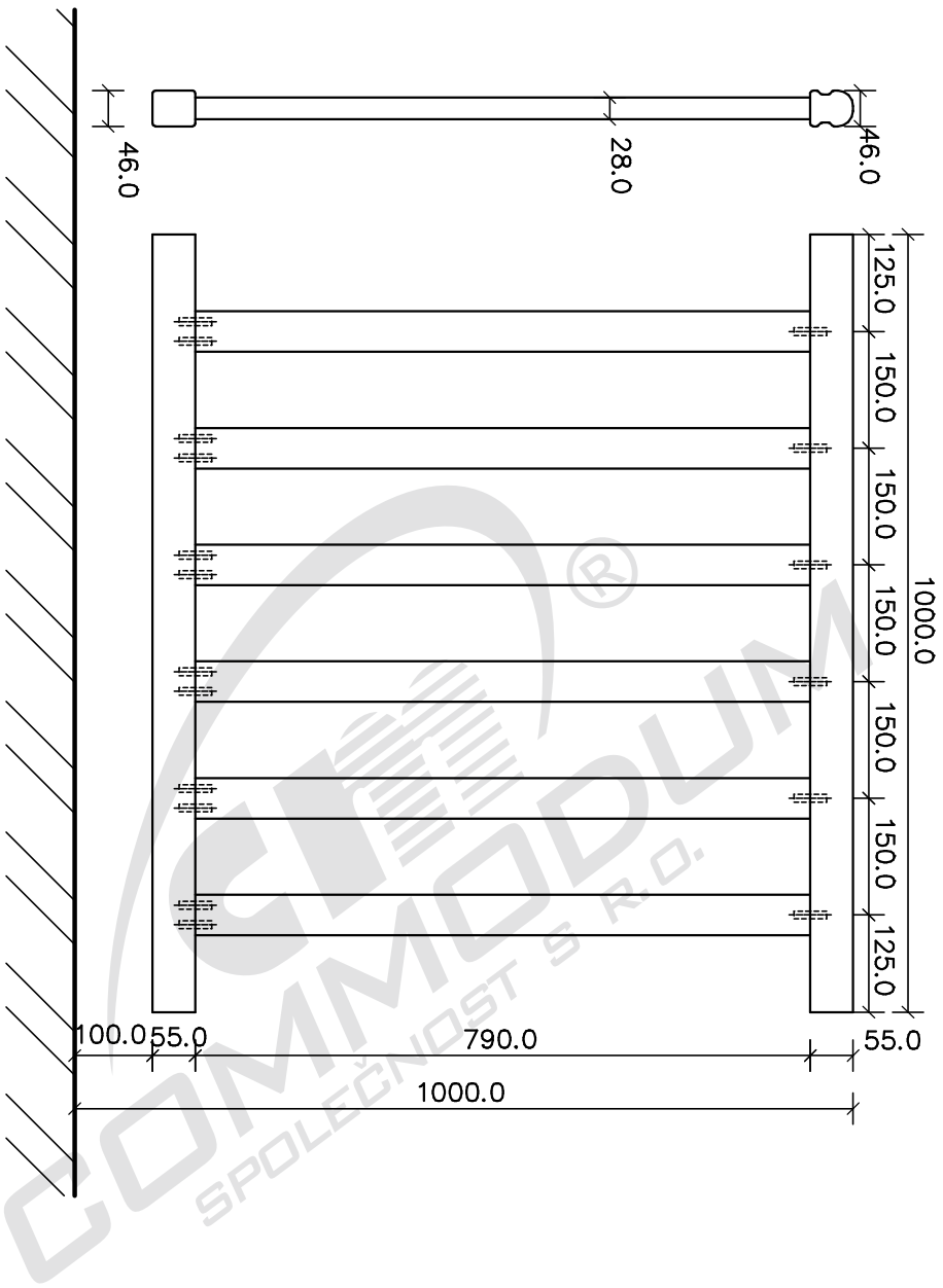
Galeriegeländer – Standardfüllung – Länge 1000mm +
